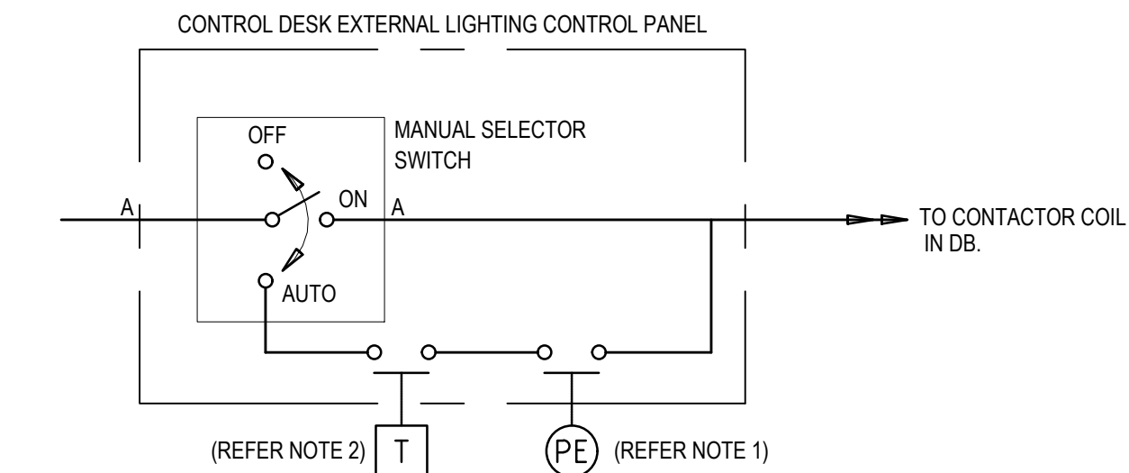
EXTERNAL LIGHTING TIME SWITCH / PE CELL CONTROL SCHEMATIC SCALE: N.T.S.
